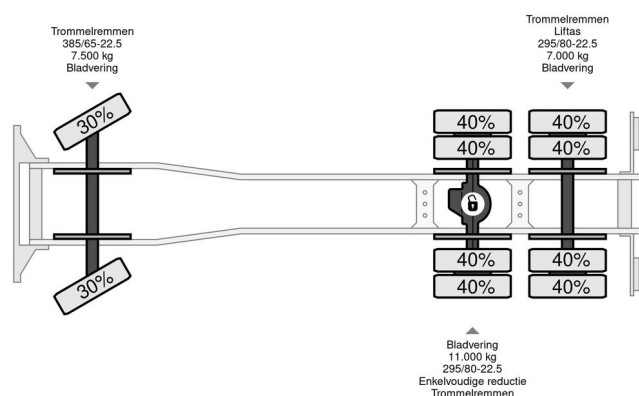
DAF XF 95.380
