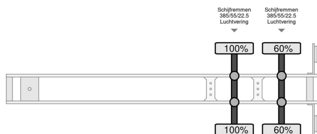
Fliegl SZS300 - 2015 - Container chassis
