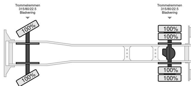
Mercedes-Benz 1620
