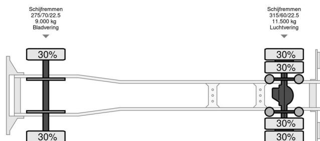
Scania G380 G380 - Schade - Damage - Schäden
