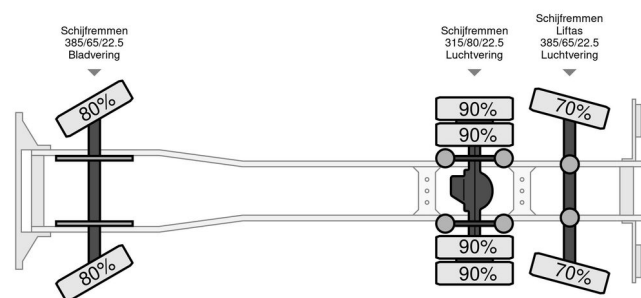
Volvo FH 480 FH 480
