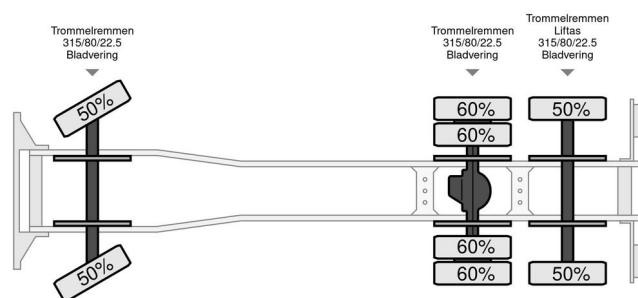
Scania R143-420 V8 Hiab 330-5 - JIB 90
