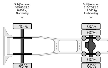
Scania R520 R520
