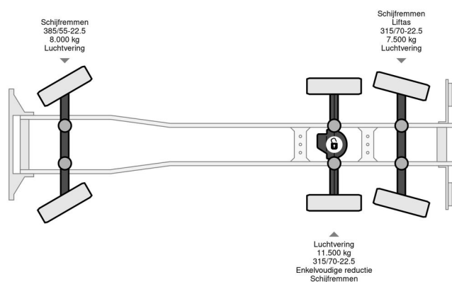
Volvo FH 13.500 FH5 500 4 Deks Pezzaioli compleet
