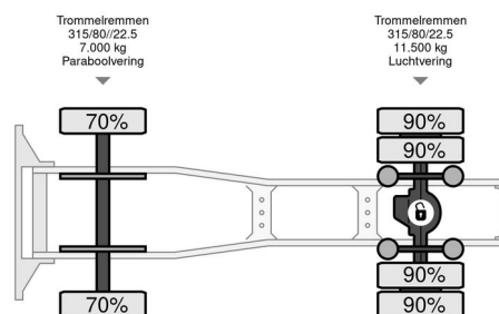
Scania R 143 MA 4X2 143 M
